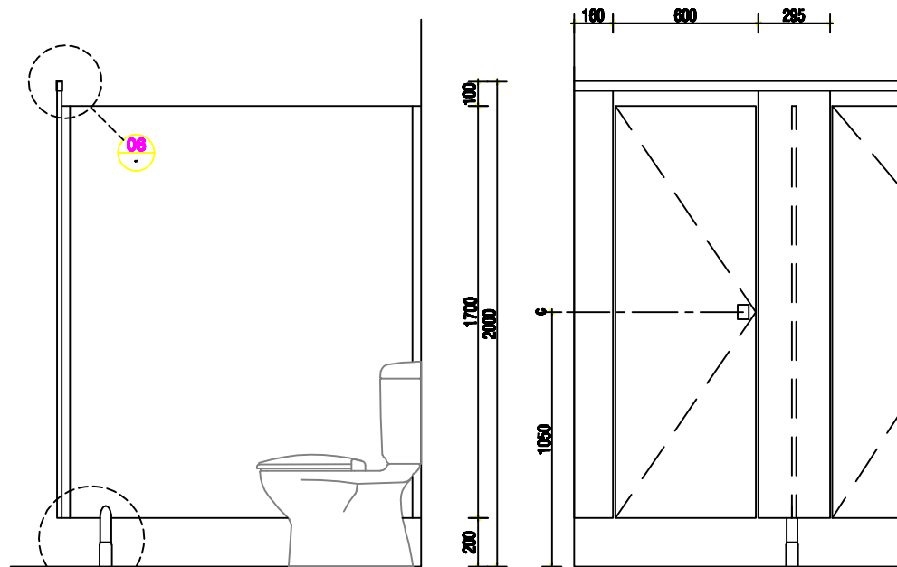
02 ELEVATION 1:10
