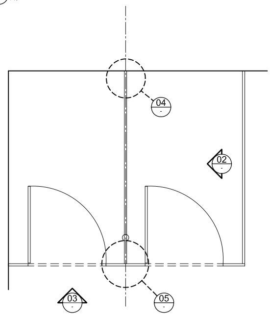
01 PLAN 1:10
