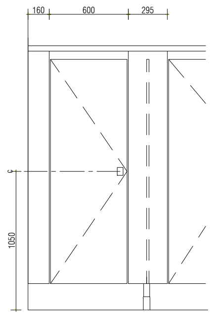
03 ELEVATION 1:10
