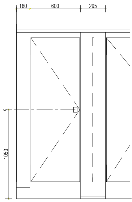
03 ELEVATION 1:10
