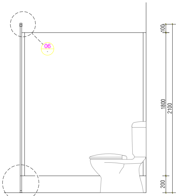
02 ELEVATION 1:10
