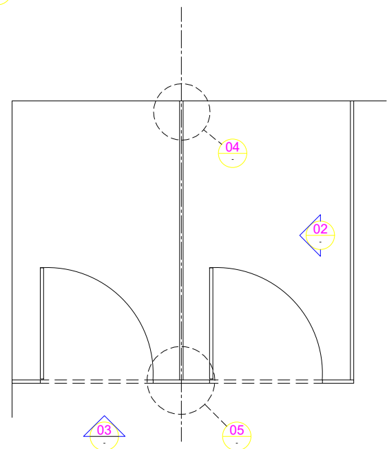
01 PLAN 1:10
