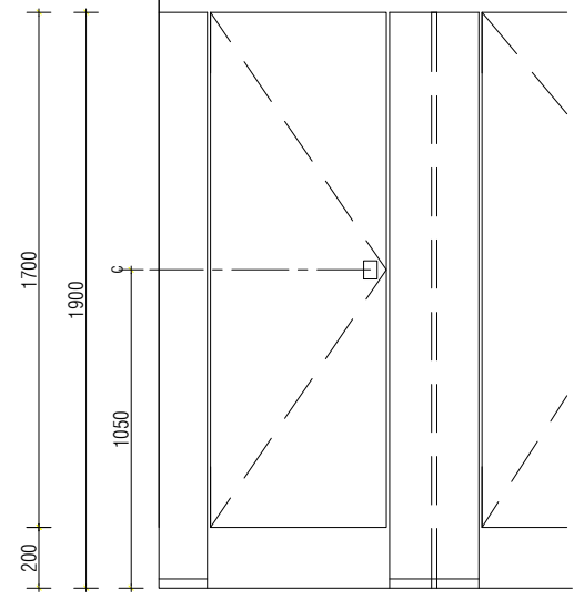
03 ELEVATION 1:10
