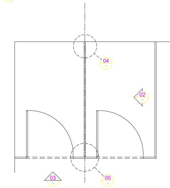
01 PLAN 1:10
