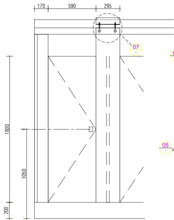
03 ELEVATION - 1:10
