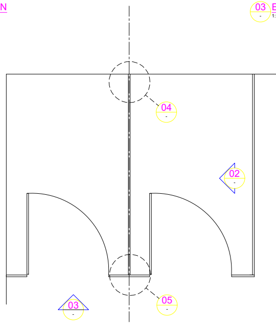
01 PLAN - 1:10
