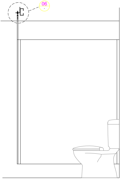
02 ELEVATION - 1:10
