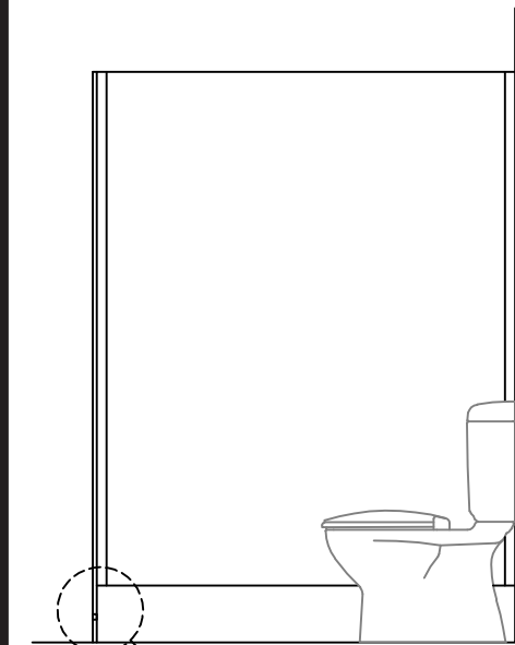
02 ELEVATION
